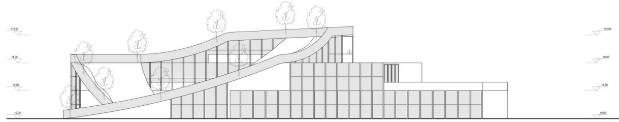
ÖN GÖRÜNÜŞ ÖLÇEK 1/200
