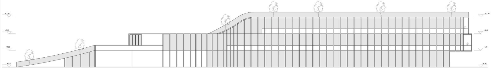
SAĞ YAN GÖRÜNÜŞ ÖLÇEK 1/200
