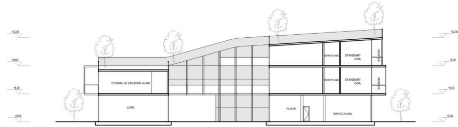
B-B KESİTİ
